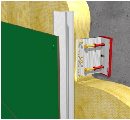
Kuitusementti / Laminaatti
