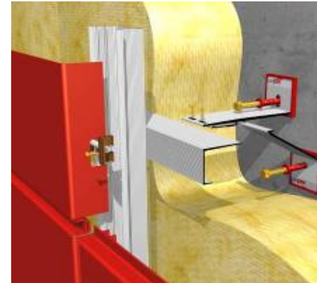
Alumiini / Komposiitti
